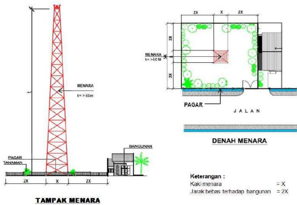
Gambar 5. Ilustrasi Jarak Bebas Menara di Atas 60 Meter terhadap Bangunan Terdekat
