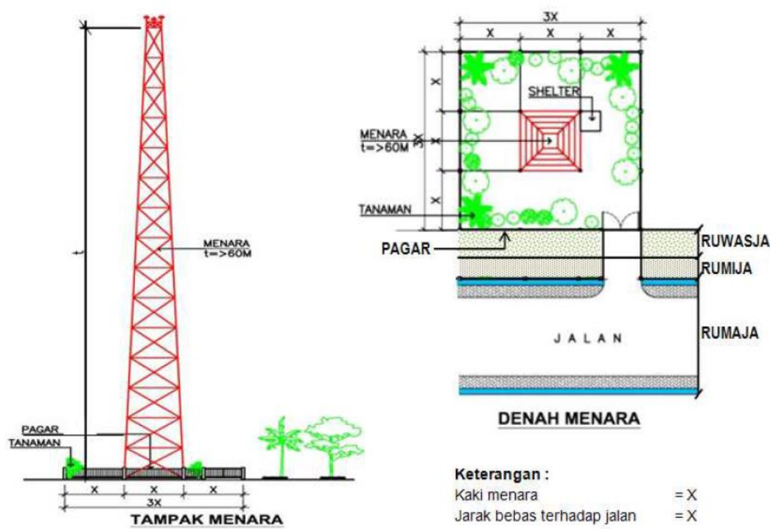
Gambar 3. Ilustrasi Jarak Bebas Menara di Atas 60 Meter terhadap Jaringan Jalan
