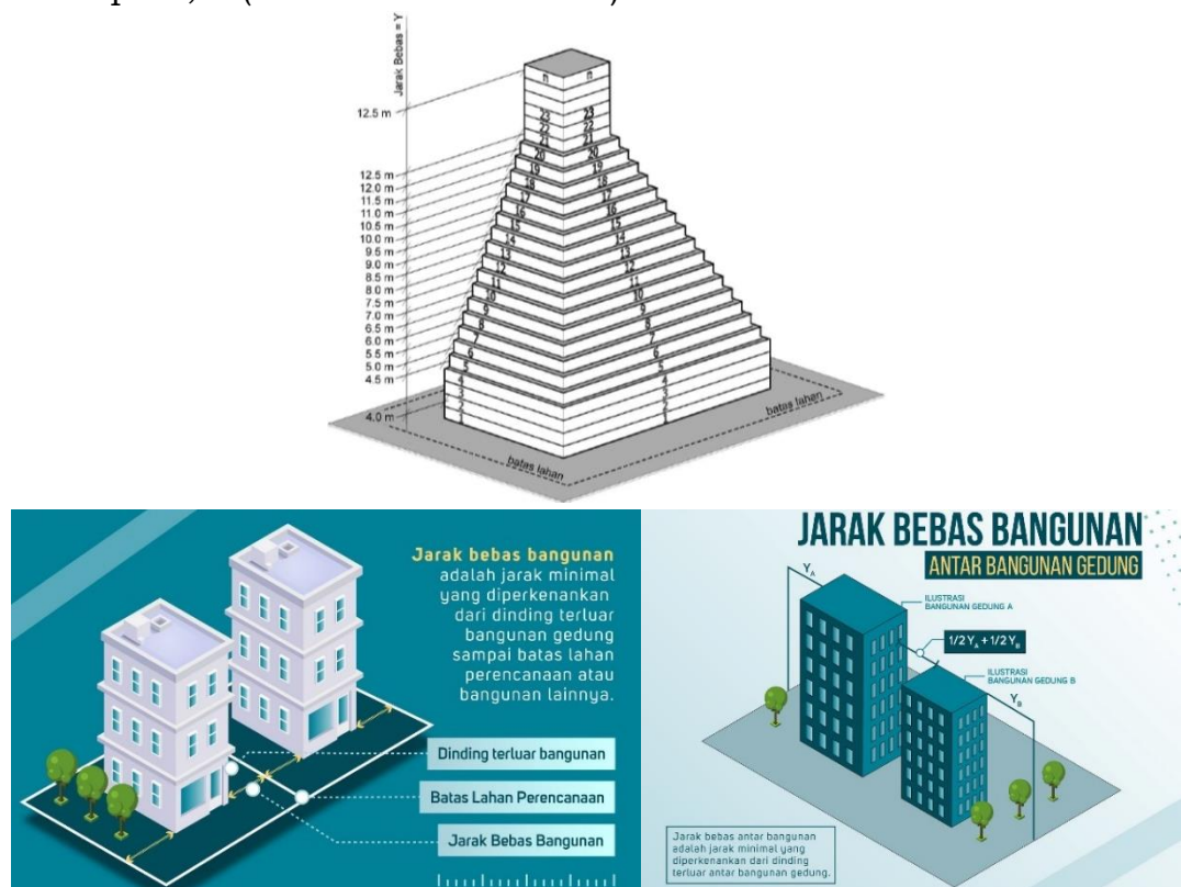
Gambar 35. Ilustrasi Penentuan Jarak Bebas Bangunan Berdasarkan Ketinggian
