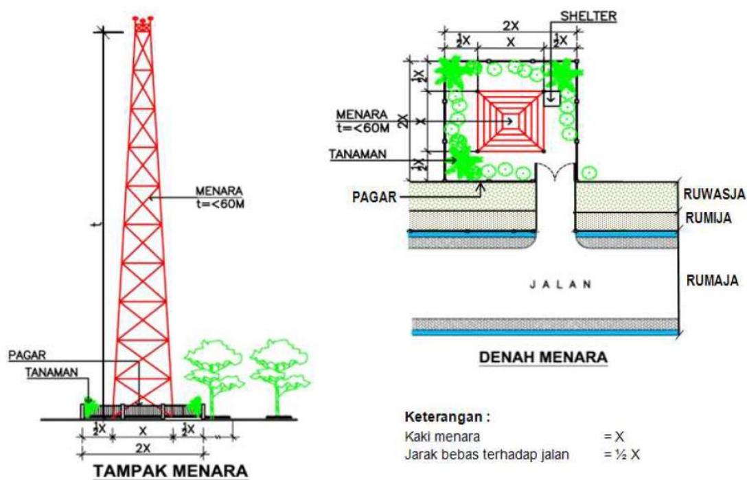
Gambar 4. Ilustrasi Jarak Bebas Menara di Bawah 60 Meter terhadap Jaringan Jalan
