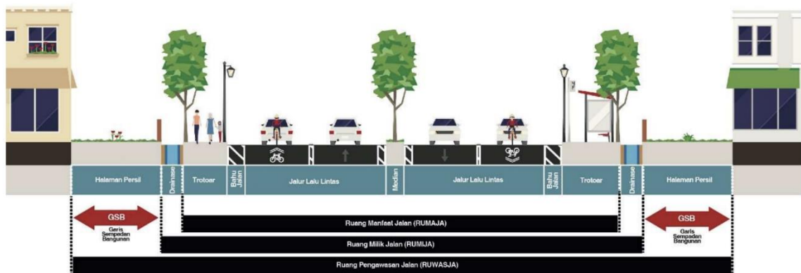
Gambar 33. Ilustrasi Penentuan Garis Sempadan Bangunan
