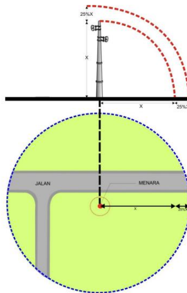
Gambar 1. Ilustrasi Radius Keselamatan Ruang di Sekitar Menara
