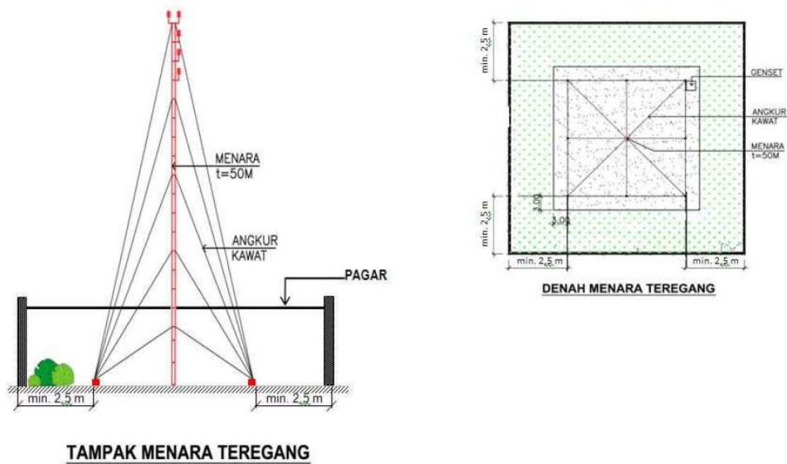
Gambar 7. Ilustrasi Jarak Bebas Menara Teregang Terhadap Bangunan Terdekat
