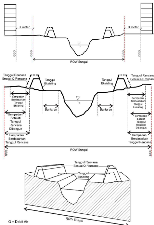
Gambar 34. Ilustrasi Penentuan Garis Sempadan Sungai
