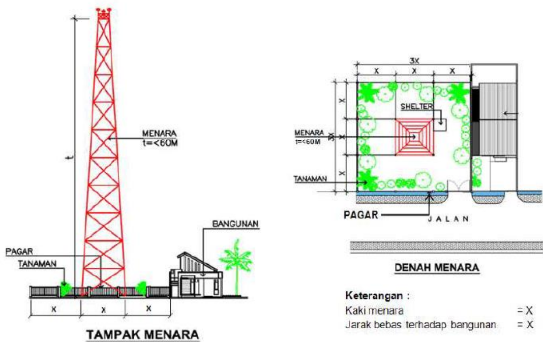
Gambar 6. Ilustrasi Jarak Bebas Menara di Bawah 60 Meter terhadap Bangunan Terdekat
