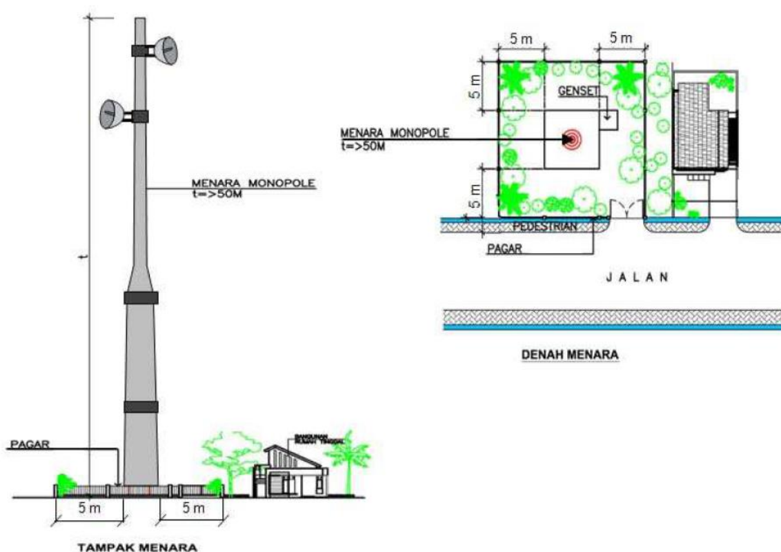
Gambar 8. Ilustrasi Jarak Bebas Menara Tunggal di Atas 50 Meter Terhadap Bangunan Terdekat
