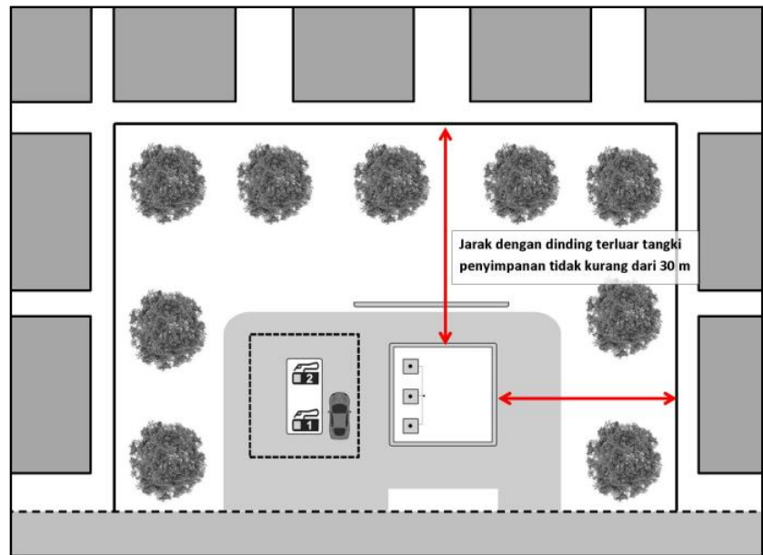
Gambar 38. Ilustrasi Penentuan Jarak Bebas Bangunan untuk kegiatan SPBU dan/atau SPBG
